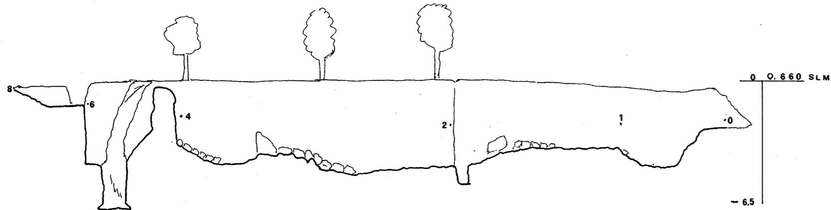
SEZ. LONGITUDINALE
